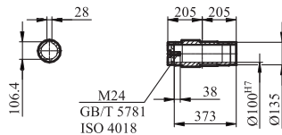
GKA/GKAZ/GKAF127输出轴
