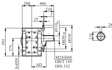
GKF127
