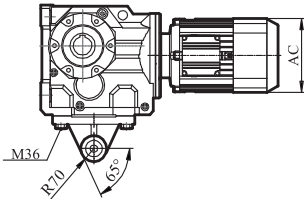
GKA/GKAZ/GKAF127输出轴
